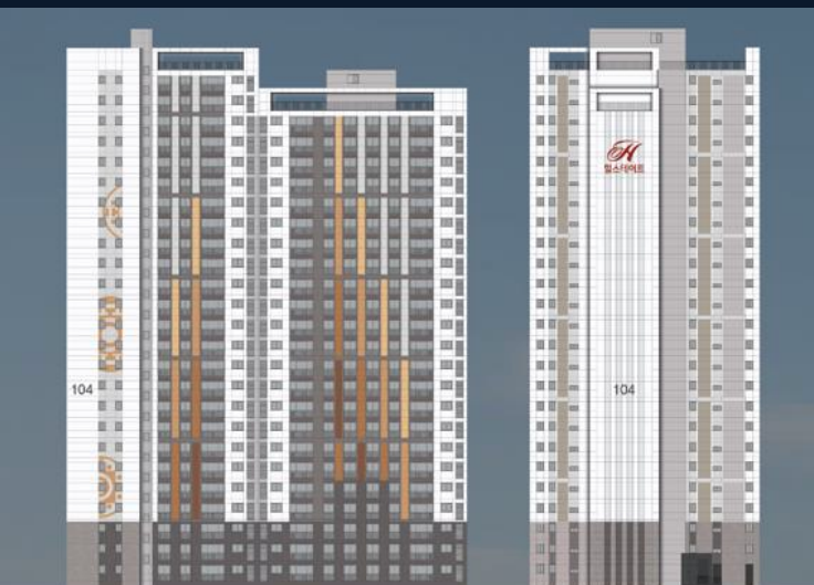
정면도
