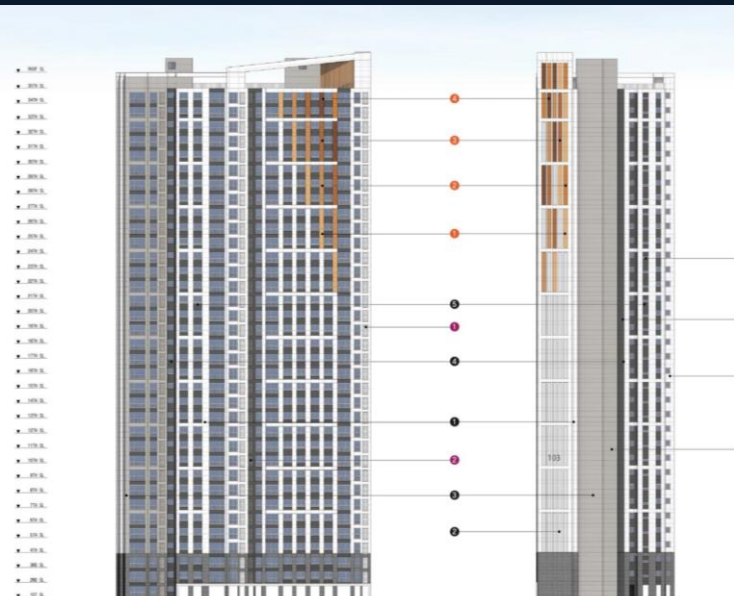
정면도
